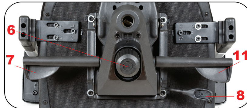
6. Geri yatma sertlik ayarı 7. Geri yatma pozisyon kilitleme ayarı 8. Oturak ileri - geri derinlik ayarı 11. Yükseklik ayarı
